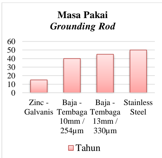
Gambar 4. Perbandingan Masa Pakai Grounding Rod.
