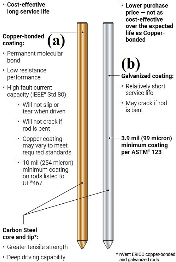
Gambar 3. Grounding Rod Material (Tembaga Lapis dan Zinc-Galvanis)
