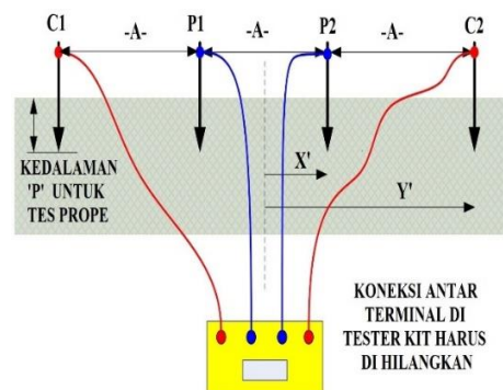
Gambar 6. Pengujian SR Metode Wenner
